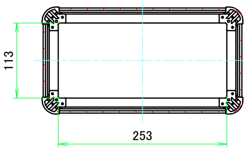
C-C ( 1 : 5.5 )
