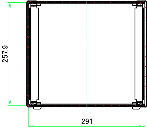
A-A ( 1 : 5.5 )
