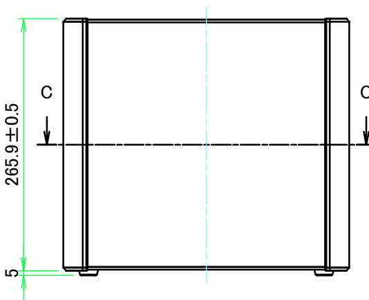
A-A ( 1 : 5.5 )
