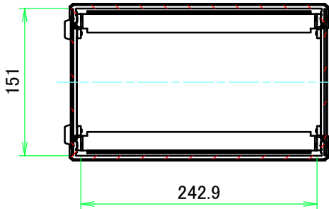
B-B ( 1 : 5.5 )
